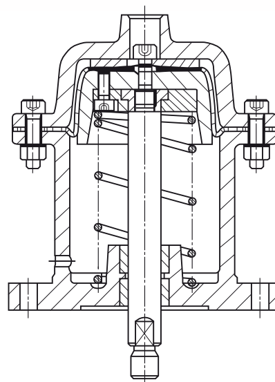
Mittelhubgerät
