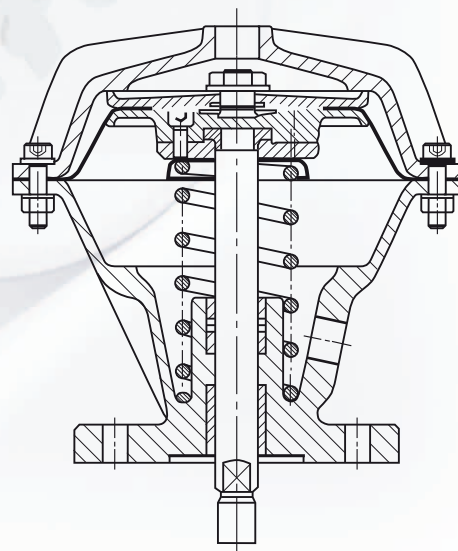
Kurzhubgerät
